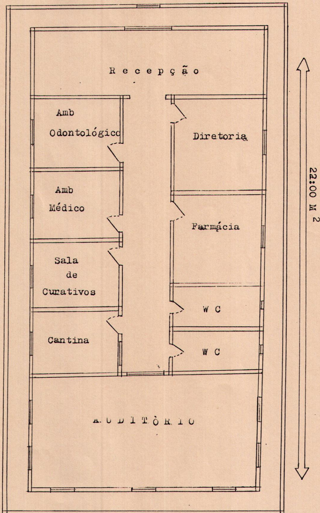
Planta baixa da Sede do Nucleo
